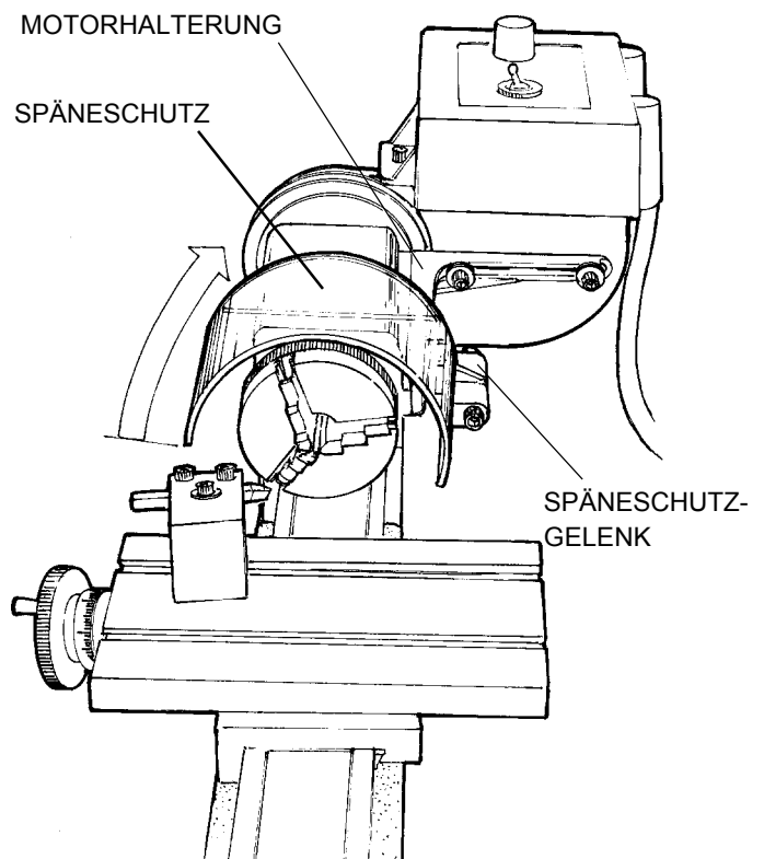
Abbildung 1: Der Späneschutz fertig montiert auf der UNITurn Drehbank. Der Späneschutz läßt sich über ein Gelenk leicht hochklappen.
